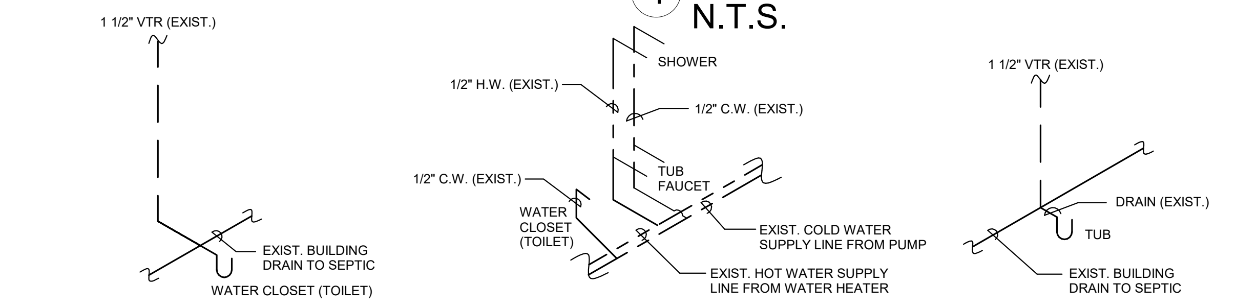
3 PLUMBING RISER DIAGRAMS N.T.S.
